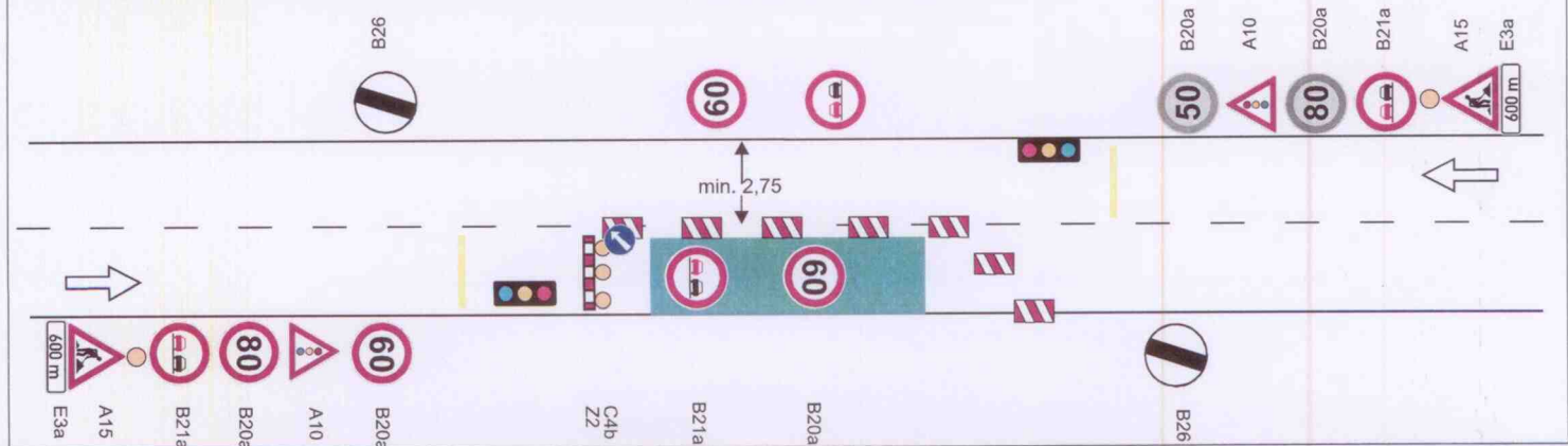
Detail pracovního místa - dle upraveného schéma C/5 bude realizováno dle vyznačených úseků.
